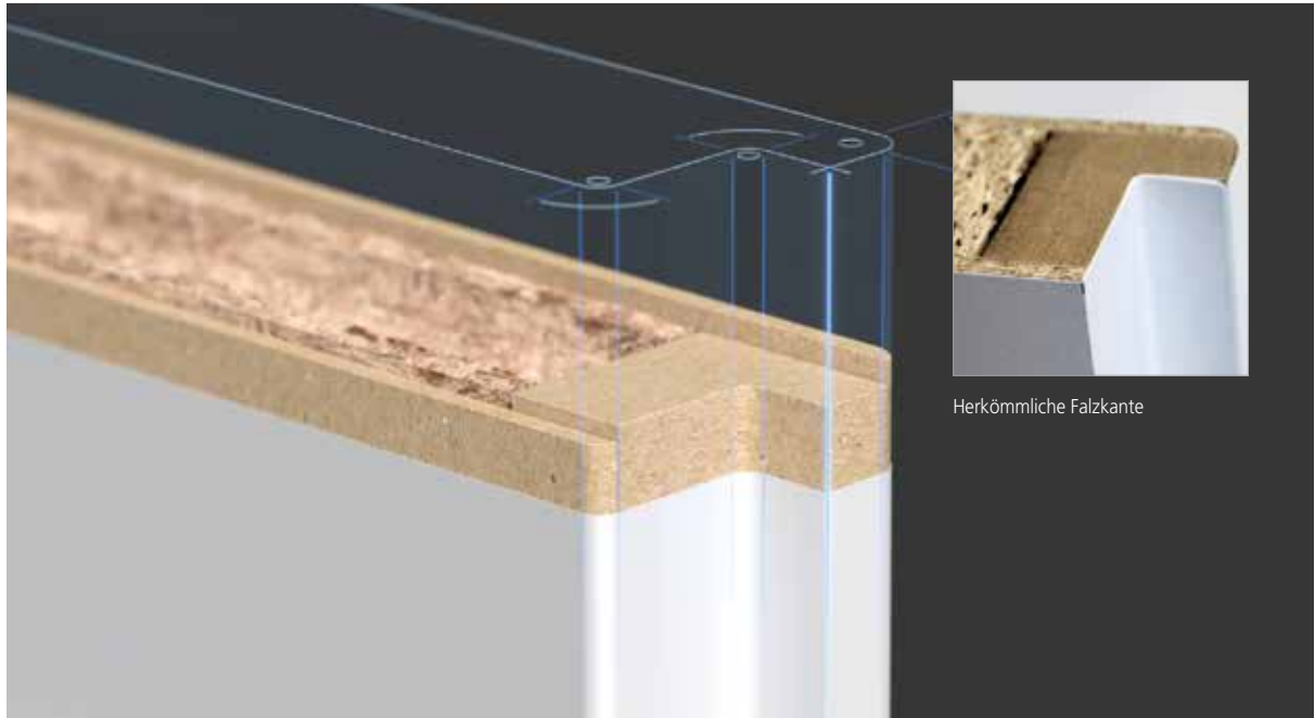
JELD-WEN Falzkante
