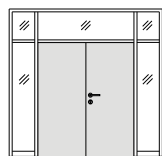
WZ7 mit Kämpfer, 2 Seitenlichtern und Oberlicht
